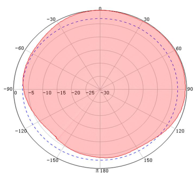
2600MHz Horizontal
